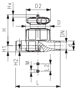
Type 515 Spigot
